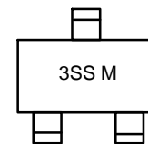
SOT-23/SUPERSOT-23 CASE 527AG
