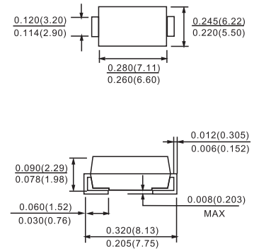
DO-214AB(SMC)
