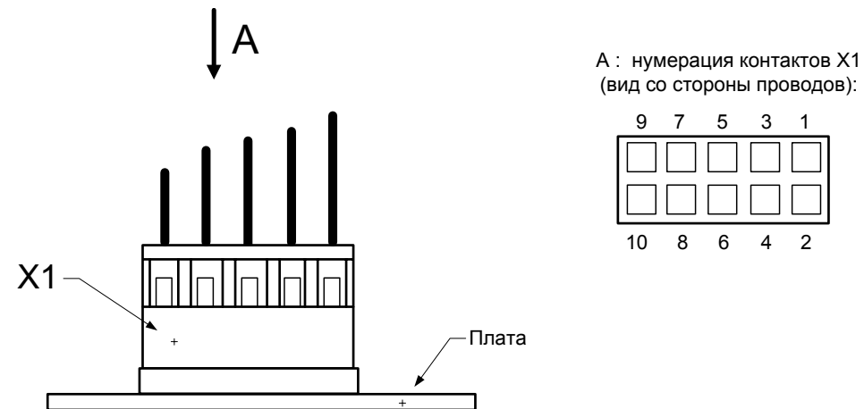
Pic.2. Нумерация контактов разъема X1
