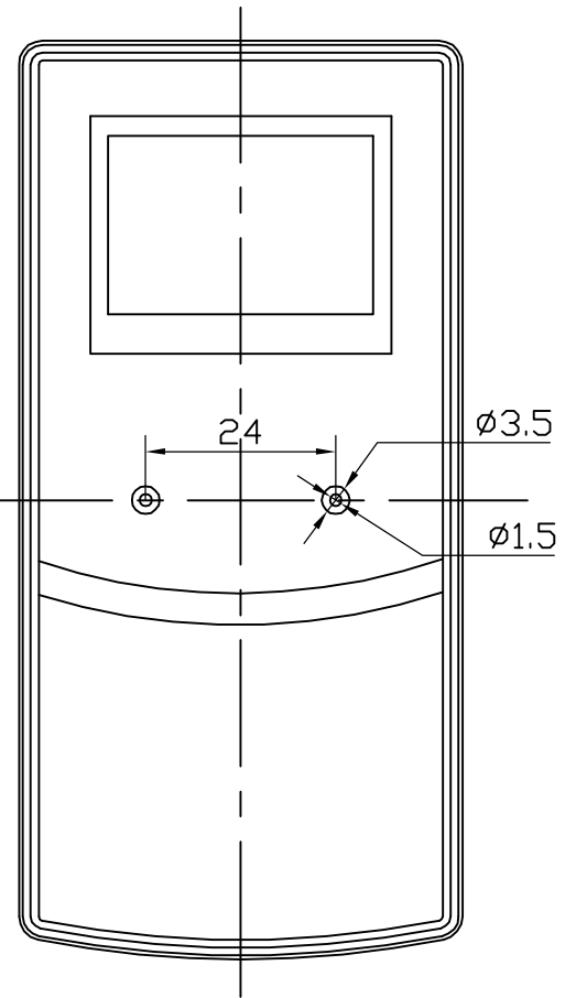
上盖底视图
