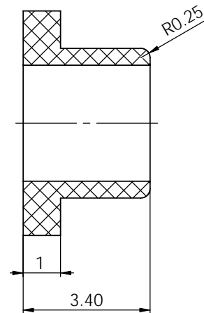
剖面 A-A
