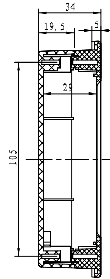
截面 B-B
