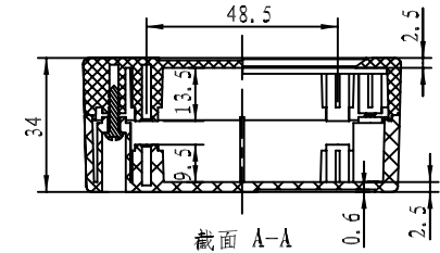
截面 A-A
