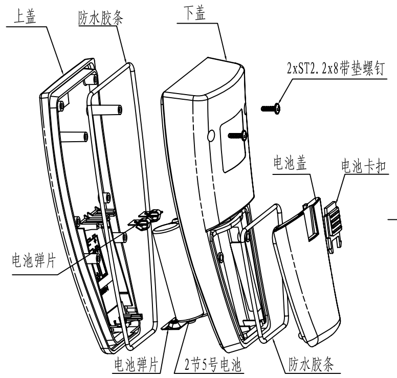
上盖线路板可按此设计
