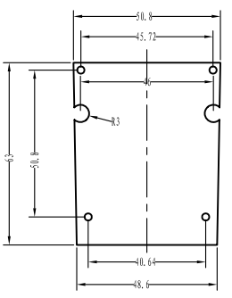
下盖线路板可按此设计
