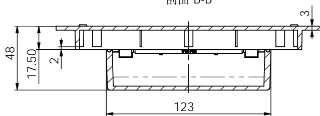
剖面 B-B
