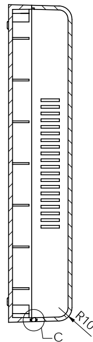
剖面 A-A
