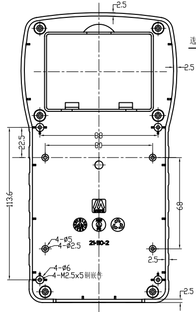
下盖正视图
