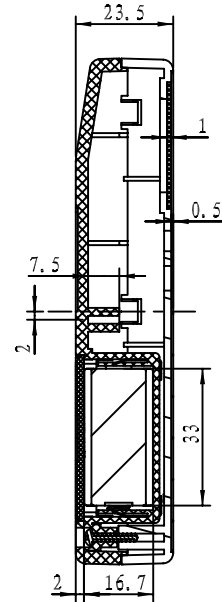
截面 A-A
