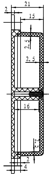
剖面 A-A
