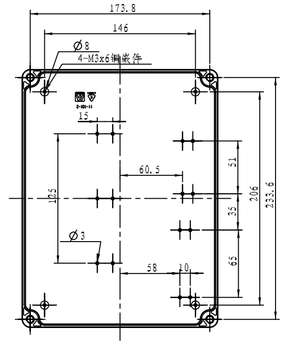
下盖正视图
