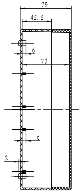
截面 A-A
