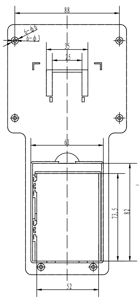
下盖底视图
