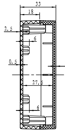
剖面 B-B
