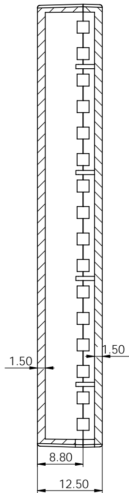
剖面 A-A
